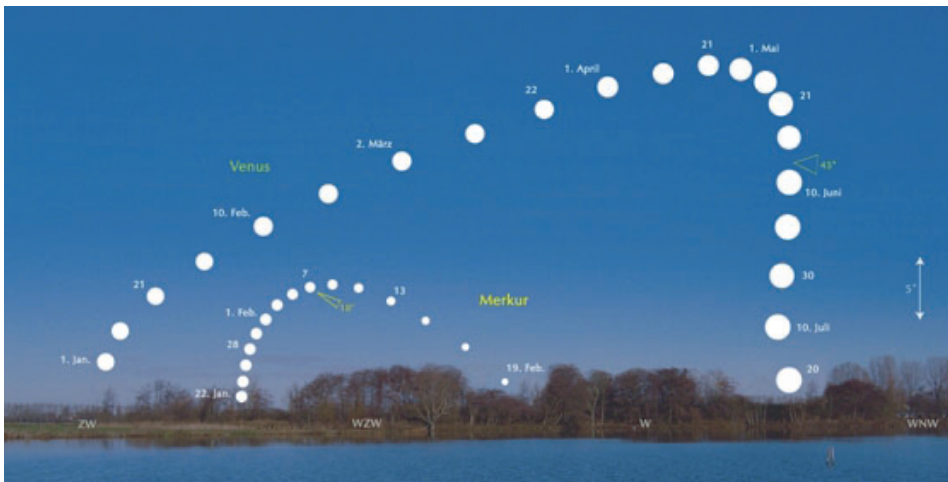
Abbildung 13: Venus am westlichen Himmel, etwa vierzig Minuten nach Sonnenuntergang, Standort Utrecht. Der Ort der Venus ist für jeden zehnten Tag abgebildet (Januar bis Juli 2007). Nach: Sterrengids 2007, De Koepel, Utrecht.
