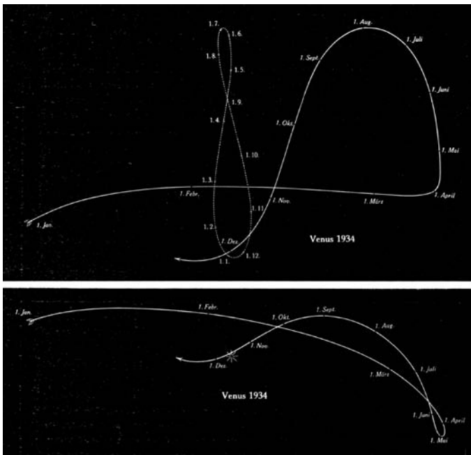
Abbildung 8: Gesamt-Bewegungs-Erscheinungen der Venus im Jahre 1934. «Die Bewegung der Venus geht im ersten Vierteljahre fast geradlinig von links nach rechts, hebt sich dann im steilen Aufstieg nach oben, nimmt in den Sommermonaten eine Höchststellung ein und sinkt dann im Herbst in tiefere Lagen hinab.» [1, S. 47]
