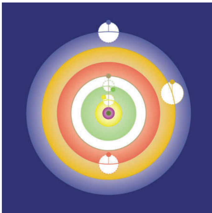
Abbildung 7: Das «dreigliedrige Weltbild» von Ptolemäus. Um die Erde (dunkelgrün) erstrecken sich Mondsphäre (violett), Merkursphäre (gelb), Venussphäre (grün), Sonnensphäre (weiss und gold), Marssphäre (rot), Jupitersphäre (orange) und Saturnsphäre (blau).
