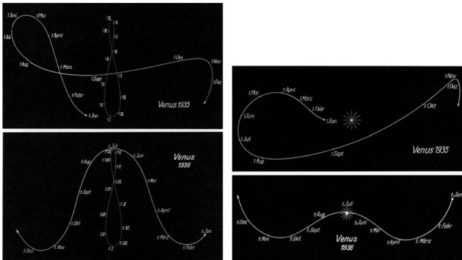
Abbildung 9: Bewegungsbilder der Venus im Jahre 1935 und im Jahre 1936 [3, S. 111 und S. 115].
