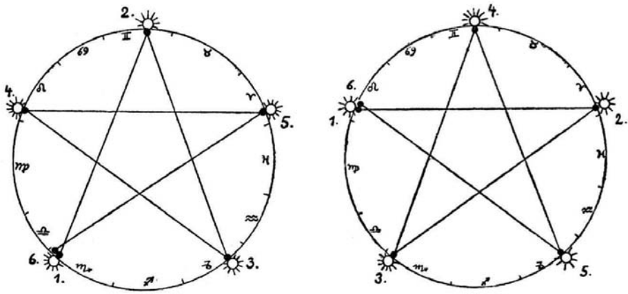
Fig. 1. Obere Konjunktionen Fig. 2. Untere Konjunktionen Verteilung und Aufeinanderfolge der Venus-Sonnen-Konjunktionen im Tierkreis. 1926—1935. 8jährige Periode.
